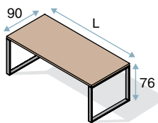
L 160 | L 180 | L 200 арт. 101 101 | арт. 101 102 | арт. 101 103
